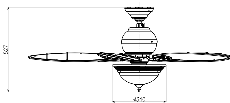
ライトキット組立外形図
